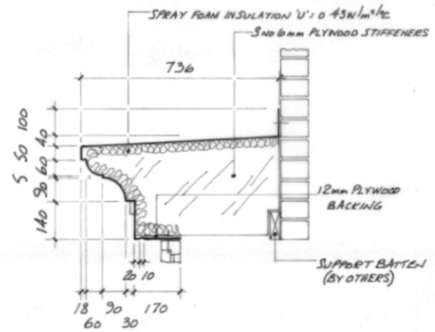
SECTION A-A 1:10
