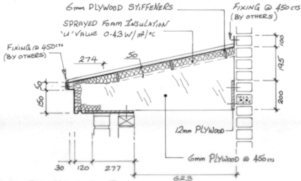
SECTION D-D
