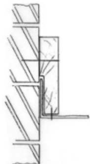
FIXING DETAIL D1
